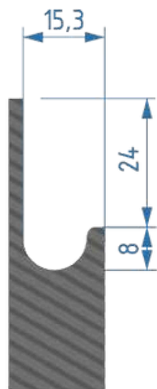
pochwył frez 38,1
