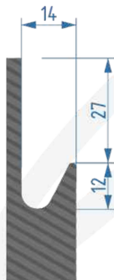
pochwył frez 45
