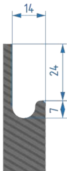
pochwył frez 34
